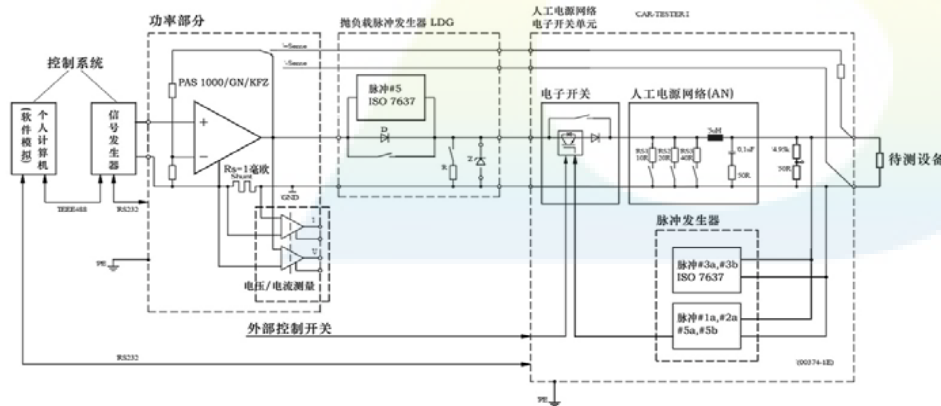
汽车电子产品测试系统框图
