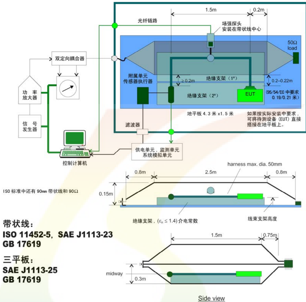
图 ISO11452-5
